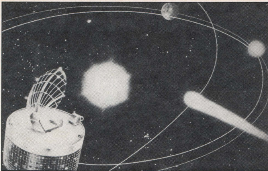
En tegners opfattelse af den japanske rumsonde Planet-A's møde med Halley's komet.
