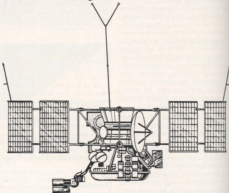
Vega rumsonderne vil »møde« Halley's komet med en hastighed på 280 km/sek.
