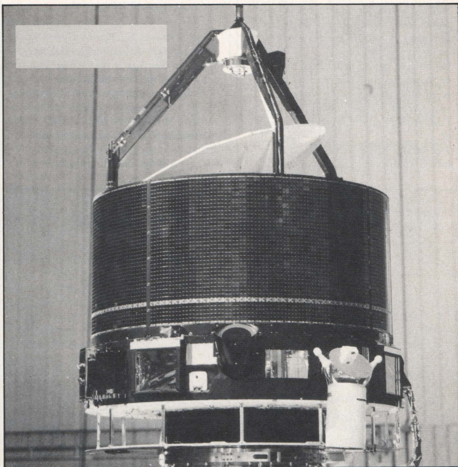
ESA kometsonden Giotto er opsendt i juli med kurs mod Halley's komet.
