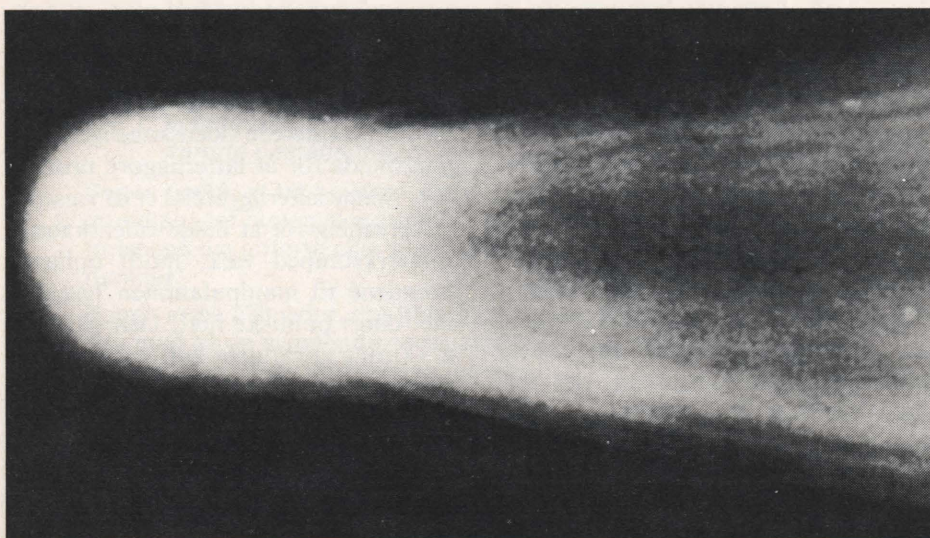
Halley's komet. Billedet stammer fra 1910.
